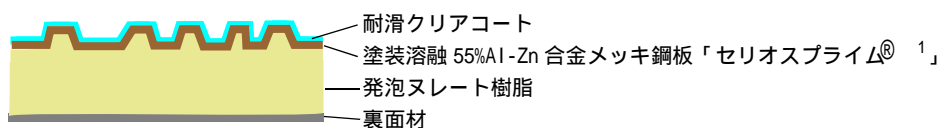
図1. 製品構成
