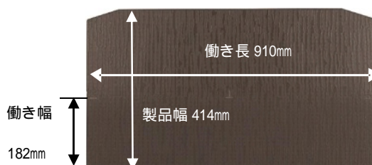
図2. 製品形状
